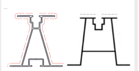
Güneş Paneli Montaj Profili H: 70
